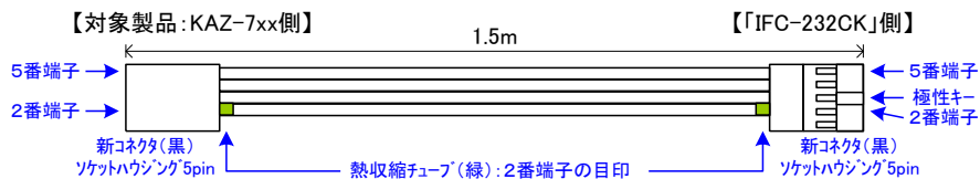
代替「通信ケーブル:CPS-IF5MCPB」外観図
