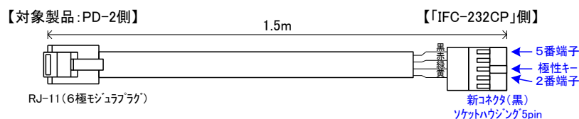
代替「通信ケーブル:CPS-IF5MCPB」外観図
