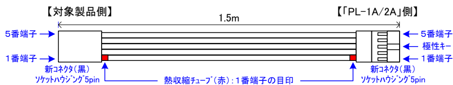
代替「通信ケーブル:CPS-PL5MCB」外観図
