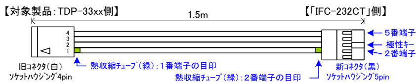
代替「通信ケーブル:CPS-IF5MCKB」外観図
