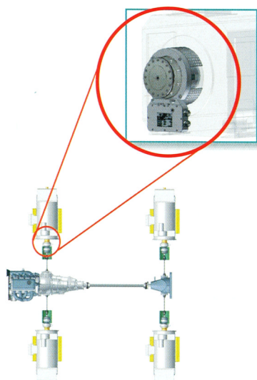
GIF製 トルクフランジ
