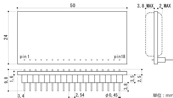
FUV-H16, FUD-H16-SPI (水平取付タイプ)
